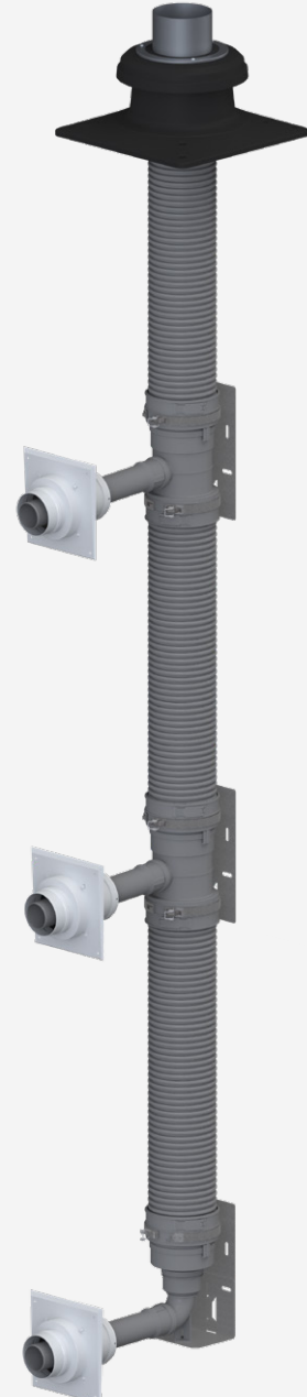
MultiFlex Gemeenschappelijke rookgasafvoer (aftakkingen 60 mm) • 100 mm MultiFlex-systeem: drie tot vier verdiepingen mogelijk • 130 mm MultiFlex-systeem: vijf tot zes verdiepingen mogelijk
